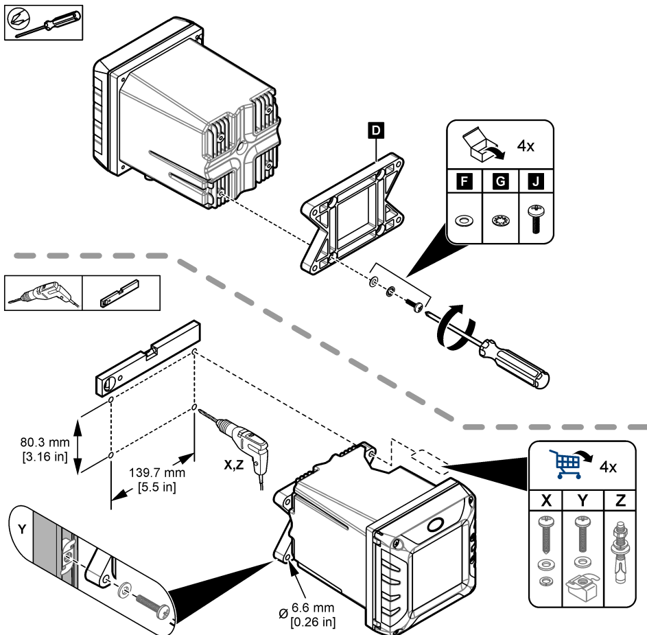
Abbildung 3 Wandmontage
