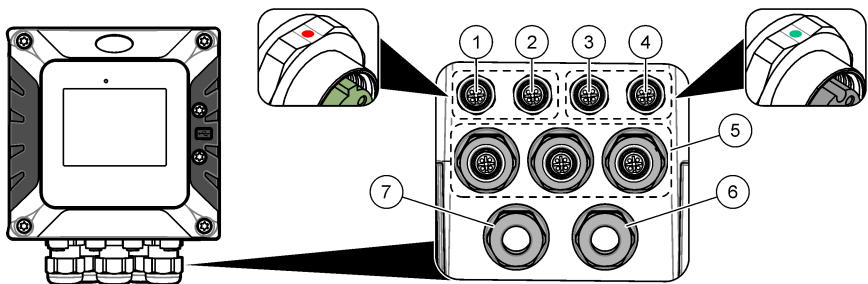
Abbildung 6 Elektrische Anschlüsse und Zugentlastungen
