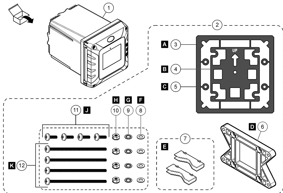
Abbildung 2 Produktkomponenten
