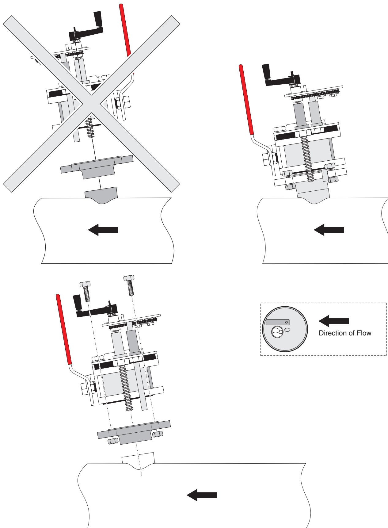
Фигура 10 Правилно положение за вграждане в тръбата
