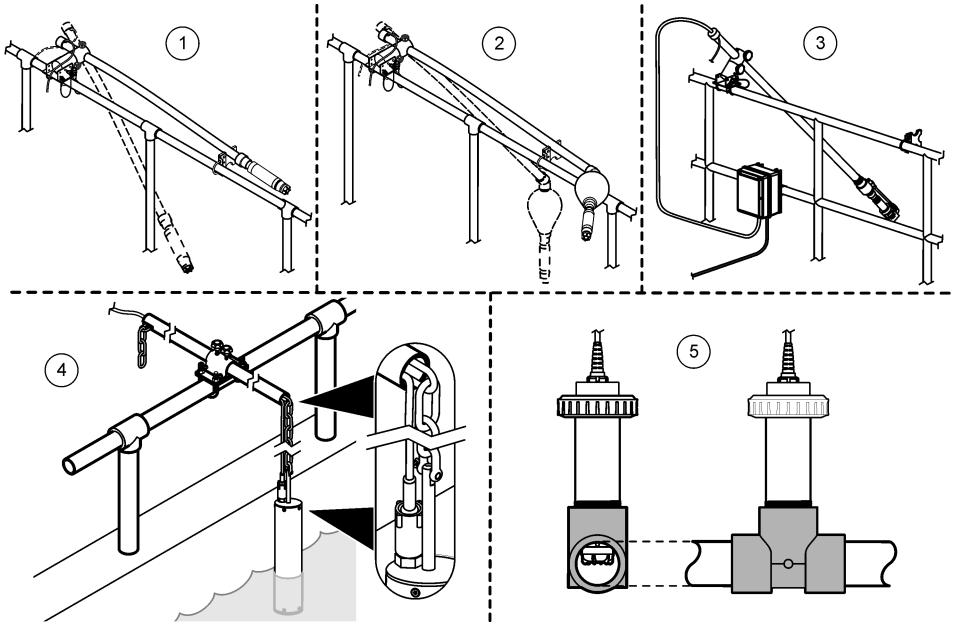
图 3 安装选项
