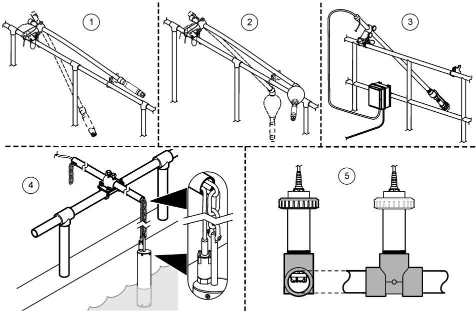
Figure 3 Options d'installation
