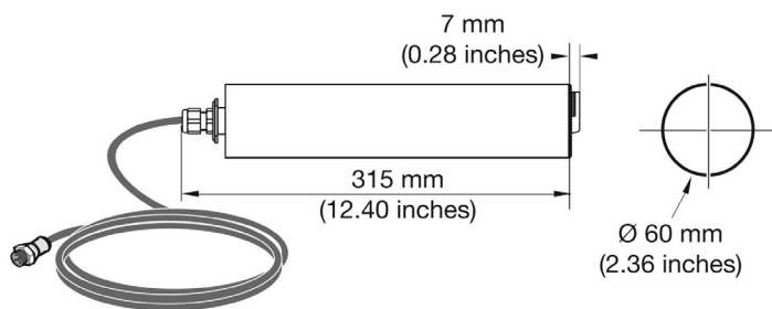
Sonde d'insertion Solitax sc
