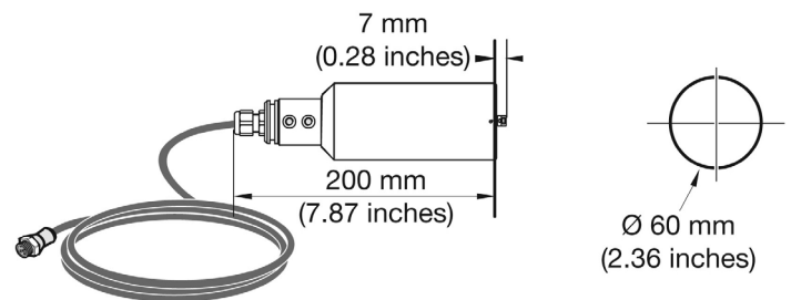
Sonde à immersion Solitax sc
