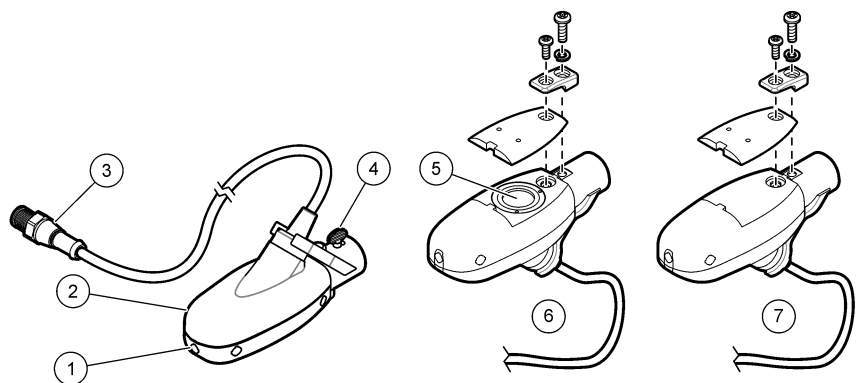
Slika 2 Komponente senzora
