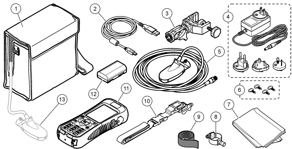
Abbildung 4 Systemkomponenten
