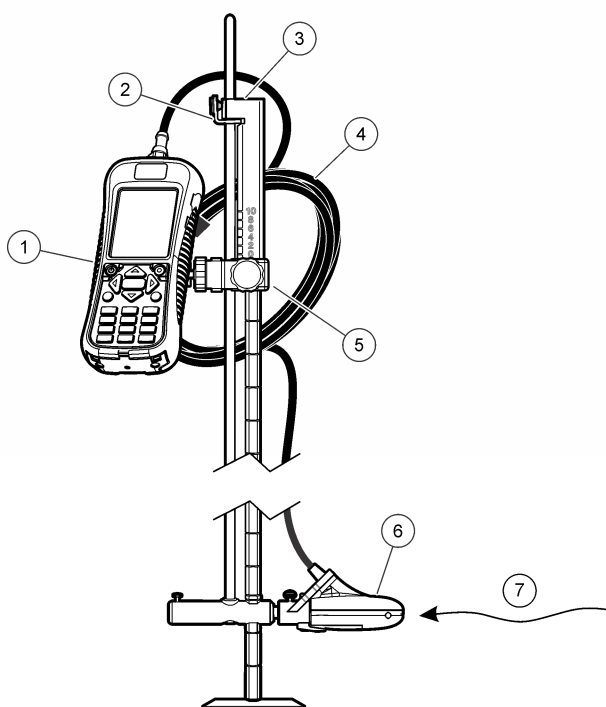
Figura 1 Componenti assemblati
