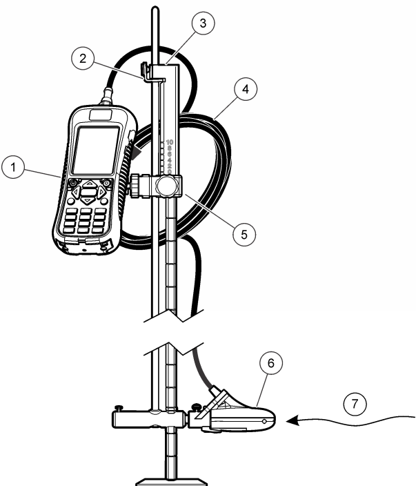
Abbildung 1 Zusammengesetzte Komponenten
