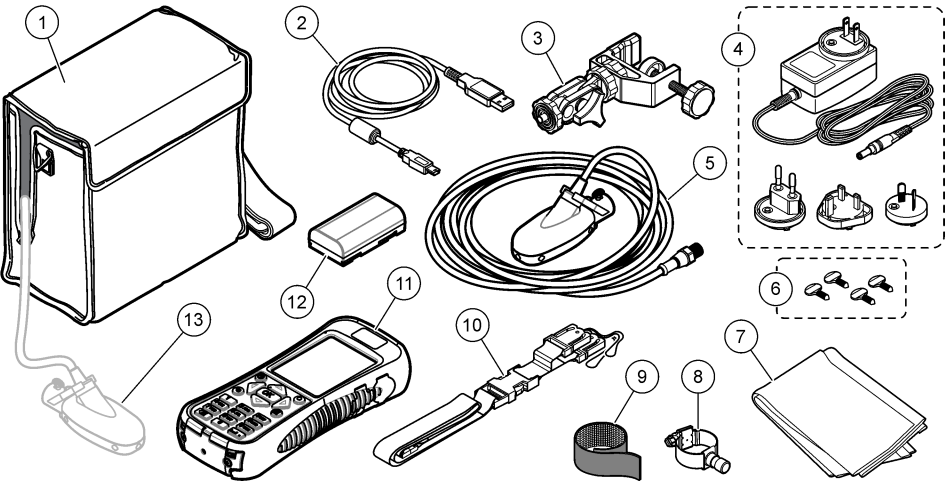
Рисунок 4 Компоненты системы
