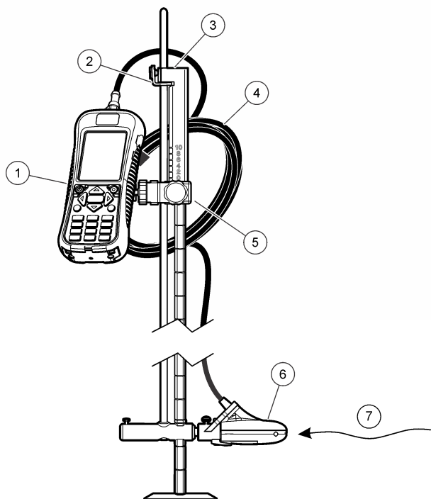
Figura 1 Componentes montados
