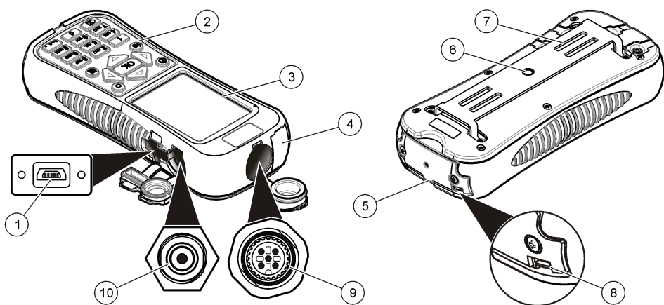
Figura 3 Componentes del medidor
