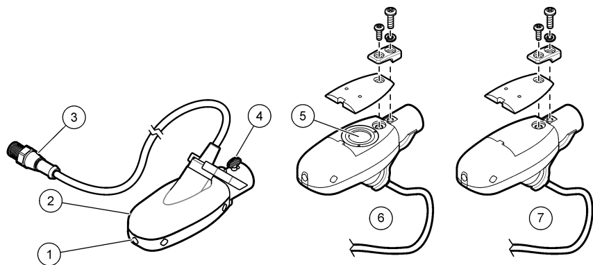
图 2 传感器组件
