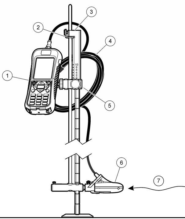
Figura 1 Componentes ensamblados
