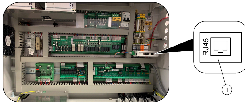
Afbeelding 7 Modbus TCP/IP-connector
