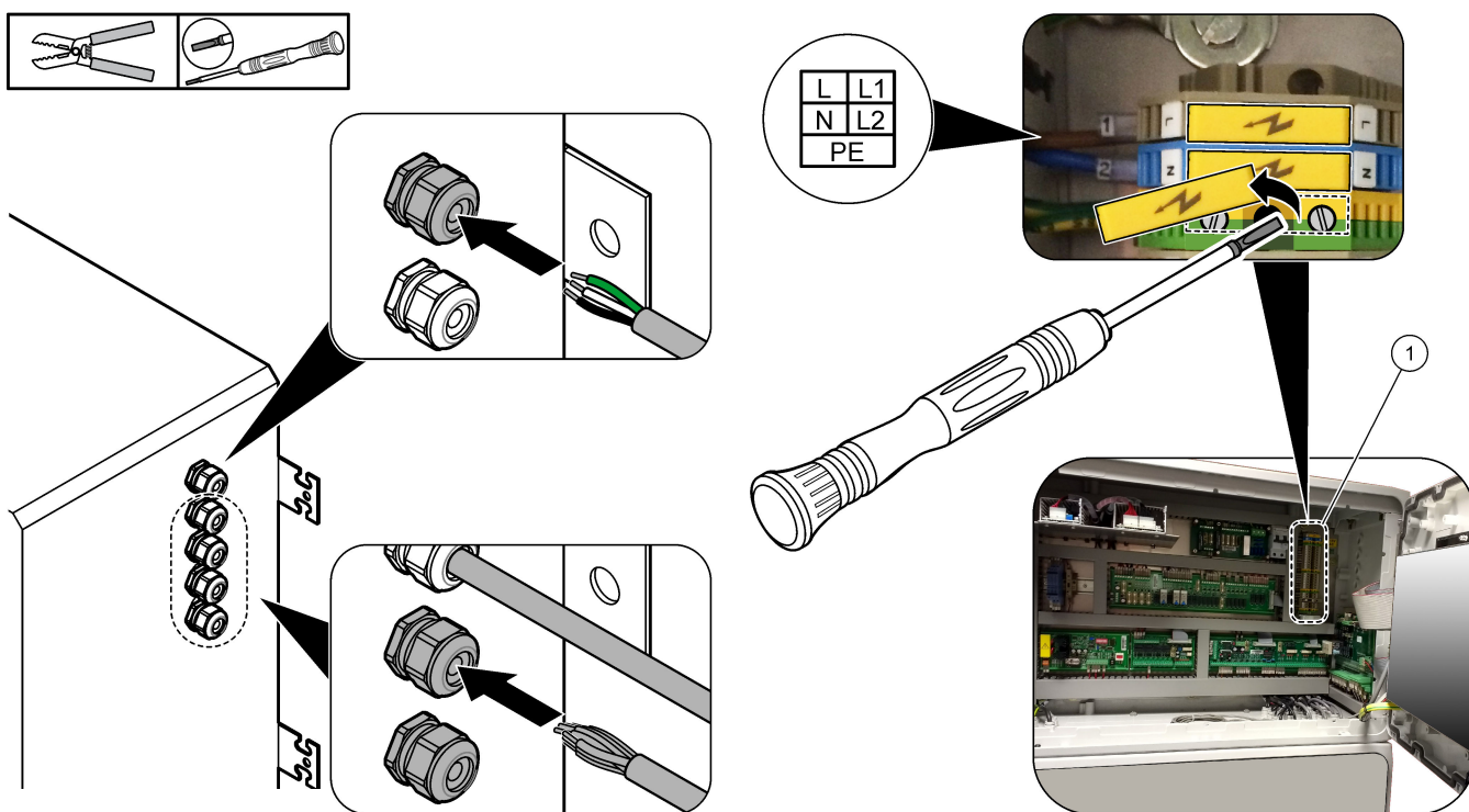
1 Voedings-, analoge uitgangs- en relaisklemmen
