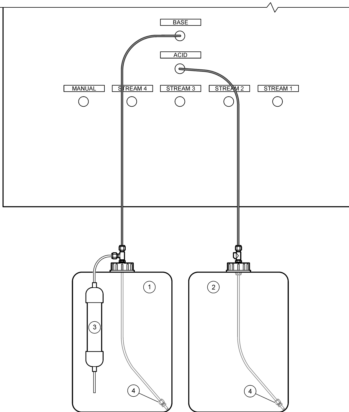
Afbeelding 15 Installatie reagens
