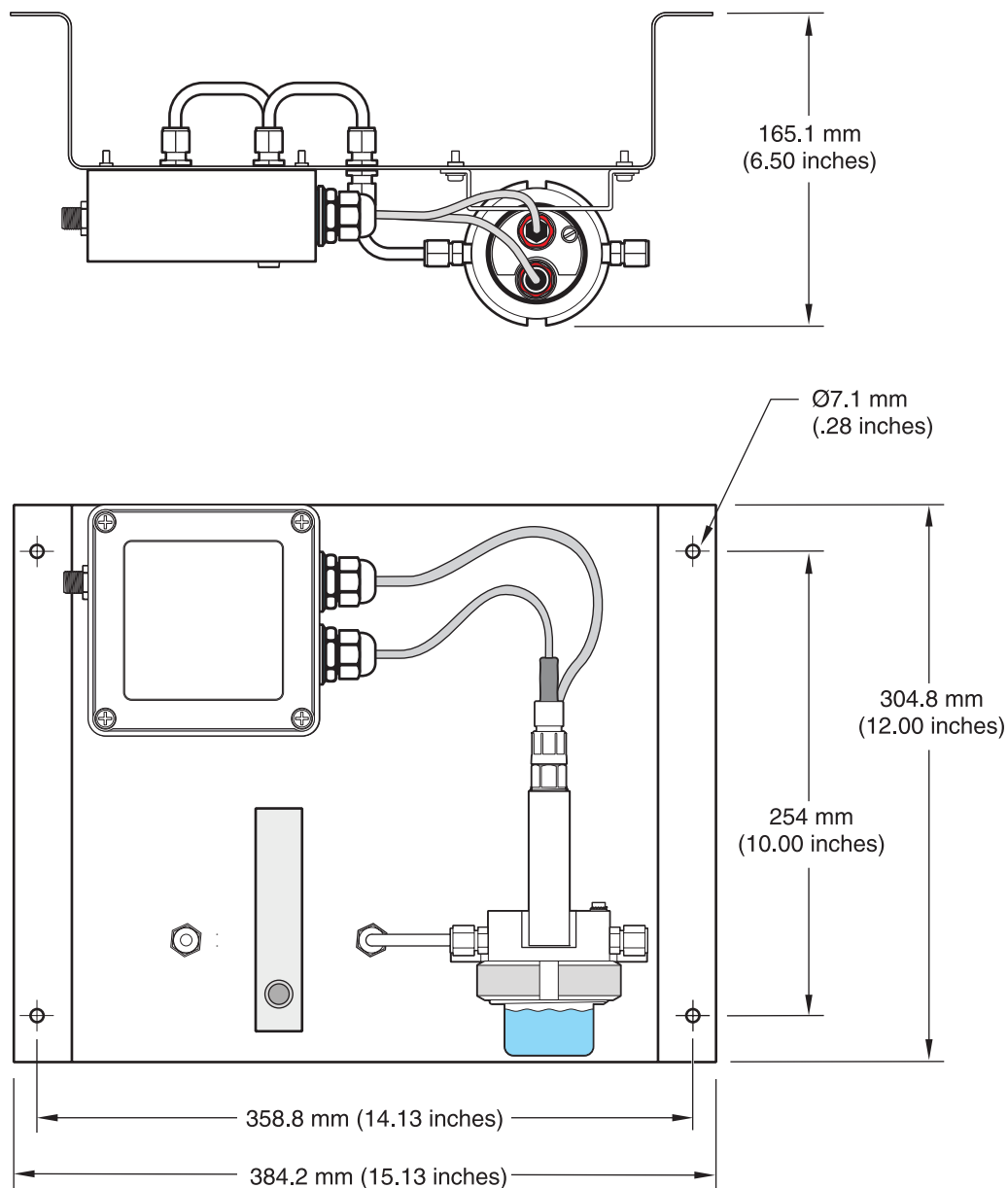
Figura 1 Dimensione di montaggio del pannello
